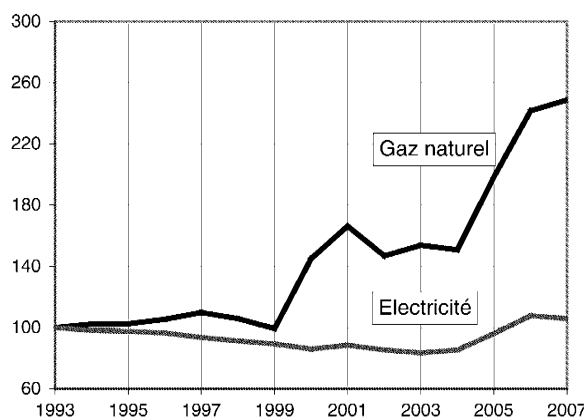
Evolution des prix de l'électricité et du gaz naturel (base 100 en 1993)
